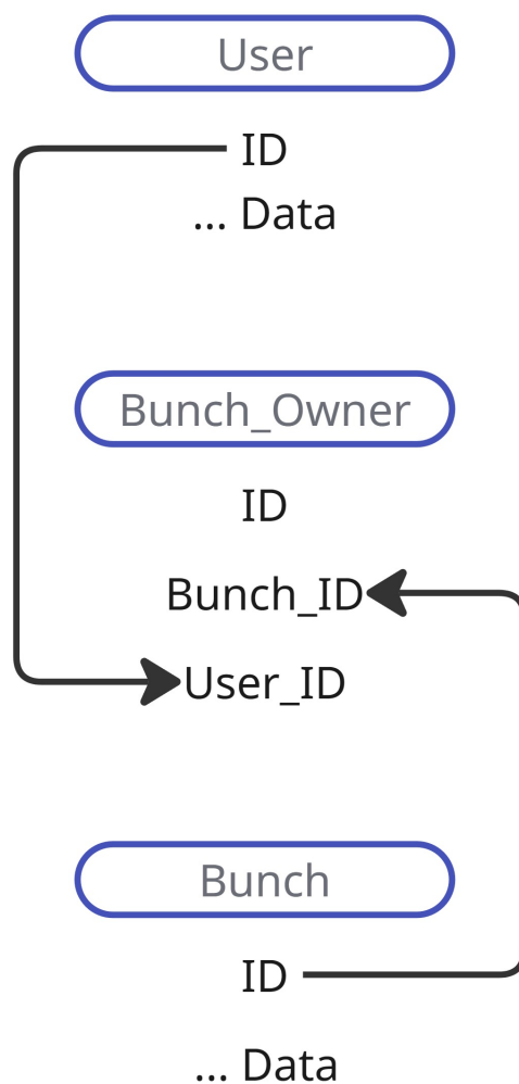
Рисунок 3. - Концептуальна модель бази даних
